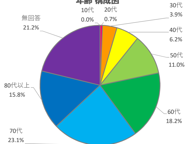
年齢 構成図
